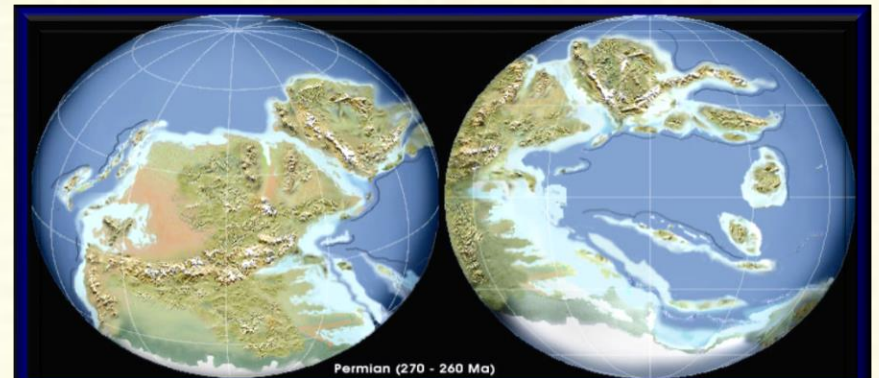
Permian (270 - 260 Ma)
